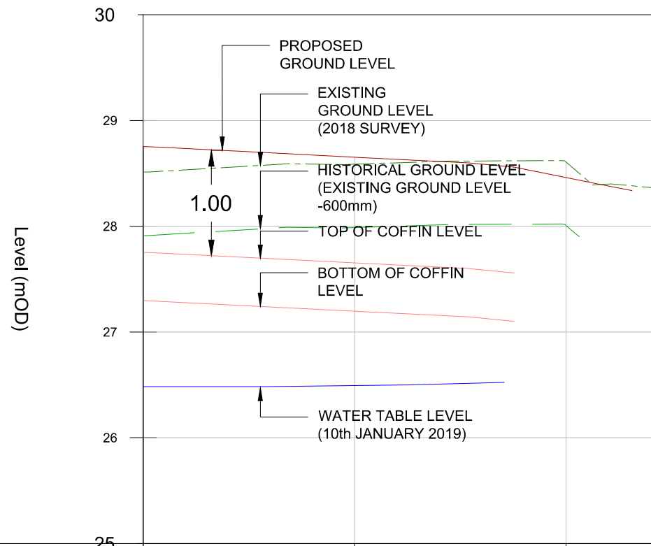
SECTION D-D - LONGSECTION SCALE: H 1:250,V 1:50. DATUM: 25.000
